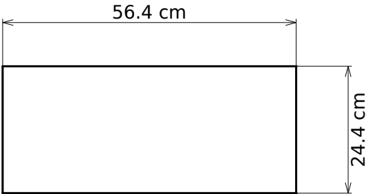
Półka, płyta MDF 18mm
